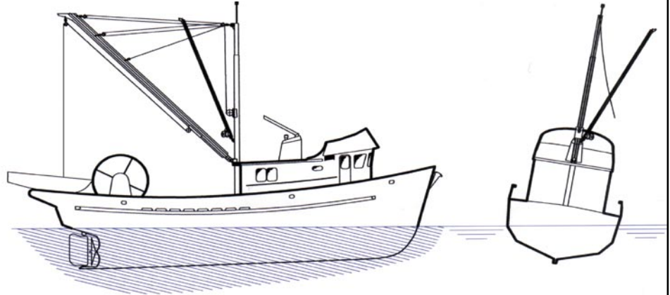
Seiner: Righting Energy Diagram
