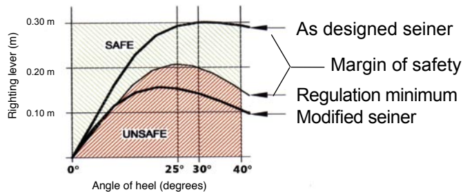
Seiner: Righting Energy Diagram
